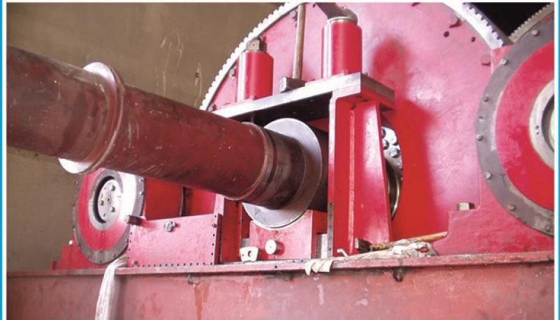
SİMETRO DİŞLİ DEĞİŞİMİ MONTAJ VE AYARLARI
