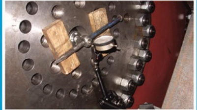
SİMETRO DİŞLİ DEĞİŞİMİ MONTAJ VE AYARLARI
